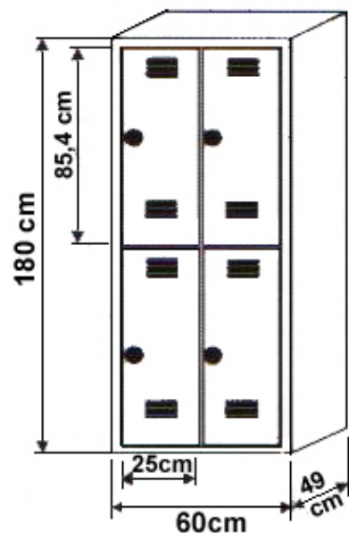
Model SU 30-2-2
